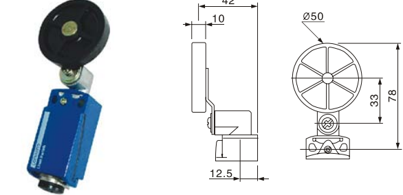
LL3XCKD 2149P16 LL3XCKD 2549P16
