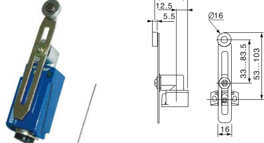
LL3XCKD2106P16 猫须式 LL3XCKD2506P16
