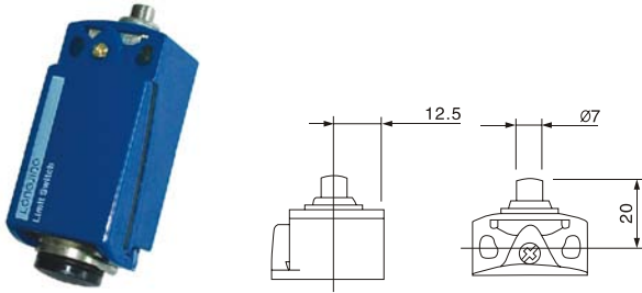
LL3XCKD2121P16 热塑滚轮水平推杆 LL3XCKD2521P16
