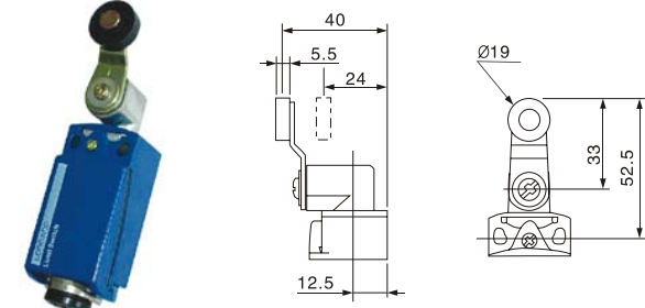
LL3XCKD2139P16 橡胶滚轮摇杆 50m LL3XCKD2539P16
