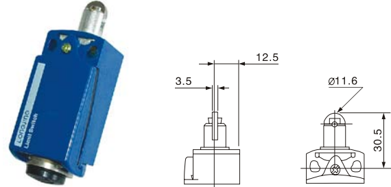
LL3XCKD21H0P16 M18 直动式 LL3XCKD25H0P16
