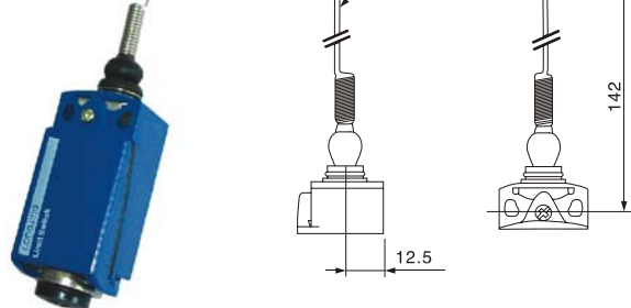
LL3XCKD2106P16 猫须式 LL3XCKD2506P16
